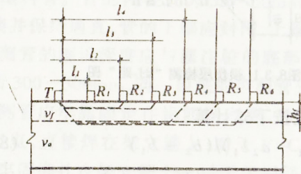
图8.2.2 检测损伤层厚度示意图
