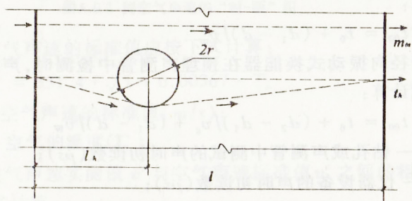
图C.0.1 空洞尺寸估算原理图
