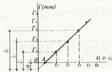
图5.2.1-1 平测“时—距”图
