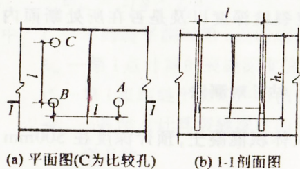
图5.4.3 钻孔测裂缝深度示意图
