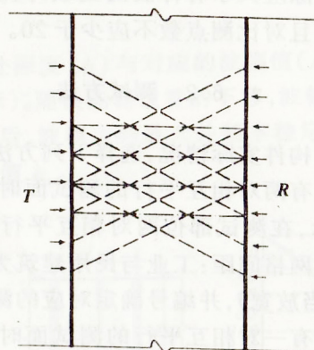
图6.2.1-2 斜测法立面图
