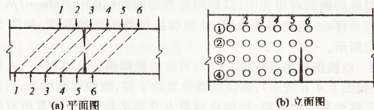
图 5.3.1 斜测裂缝测点布置示意图
