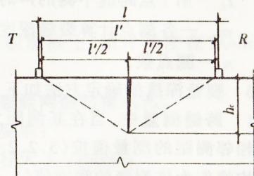
图5.2.1-2 绕过裂缝示意图
