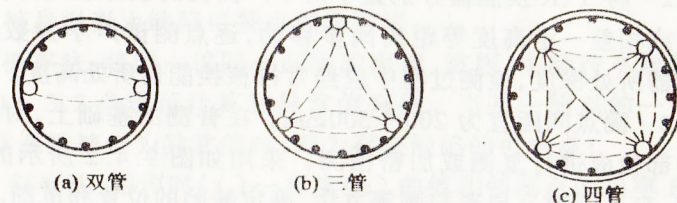
图9.2.1 声测管埋设示意图
