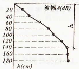
图5.4.6 h-A 坐标图
