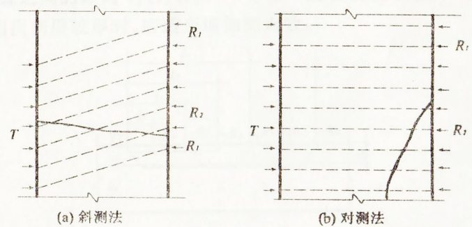
图 7.2.2 混凝土结合面质量检测示意图
