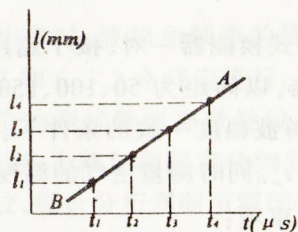
图A.0.2 测空气声速的“时-距”图
