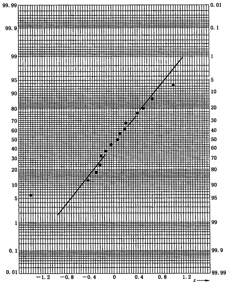
图 1 正态概率纸
