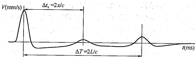
图4 缺陷桩典型时域信号特征
