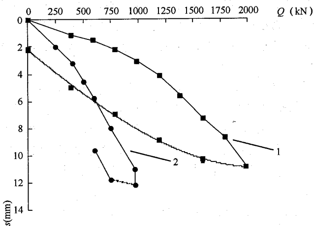
图9 静载和动载模拟的 Q-s 曲线 1—静载曲线；2—动测曲线
